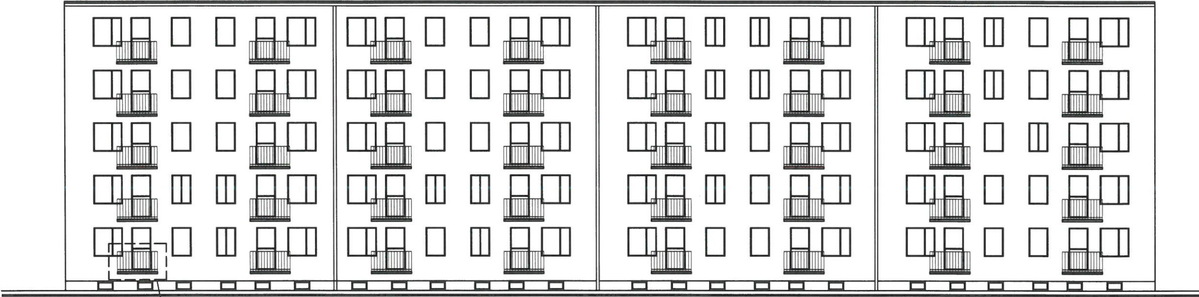
ELEWACJA ZACHODNIA BUDYNKU
